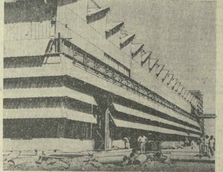
Индия. В Ранчи с дружественной помощью Советского Союза сооружается государственный завод тяжелого машиностроения. На снимке: цех металлоконструкций блока цехов для производства коксхимического и подземно-транспортного оборудования.
