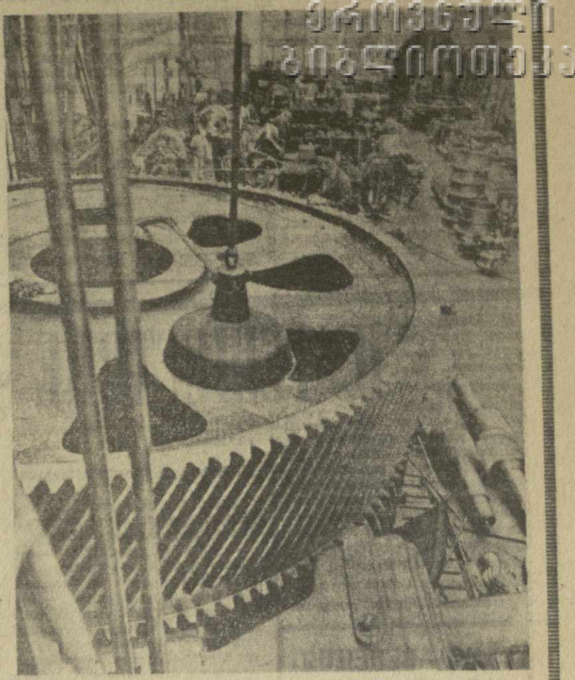
ЧССР. Западные Чехия. На Паьзенском машиностроительном заводе имени В. И. Ленина изготовлено гигантское колесо для зубчатой передачи (его диаметр — свыше четырех метров, вес — 50 тонн). Колесо является частью огромных ножиц для резки стали. Фото ЧТК—АПН.
