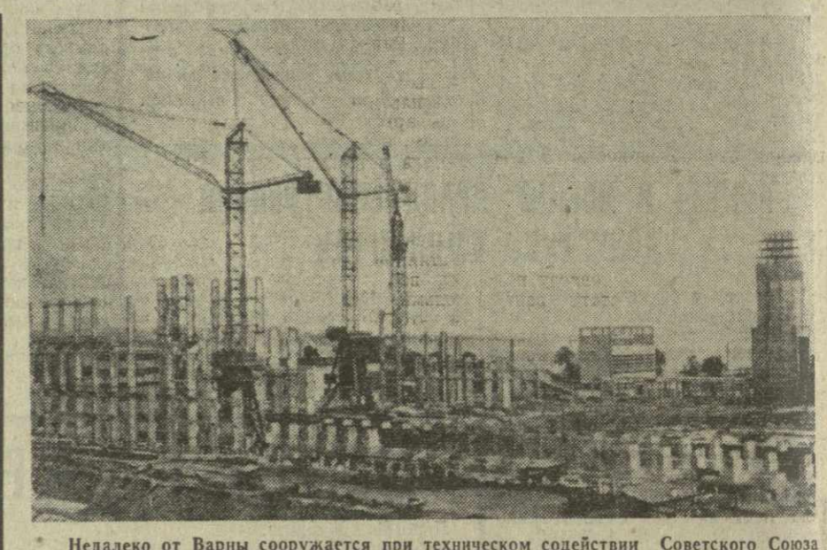
Недалеко от Варны сооружается при техническом содействии Советского Союза мощная ТЭС. Строительство станции ведется по проекту, разработанному московскими проектно-конструкторскими организациями, оборудование также поставляется советскими машиностроительными заводами. По предварительным расчетам, ТЭС «Варна» будет производить 4 миллиарда киловатт-часов электроэнергии в год. На снимке: строительство ТЭС «Варна». Фото БТА—АПН.
