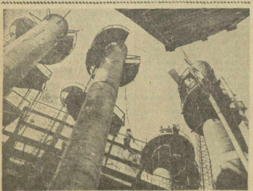
Ряд новых крупных цехов воздвигается на особо важной стройке семилетки — на Ереванском заводе синтетического каучука имени С. М. Кирова, которая объявлена ударно-комсомольской стройкой. На снимке: монтаж отделения концентрирования нового цеха завода.
