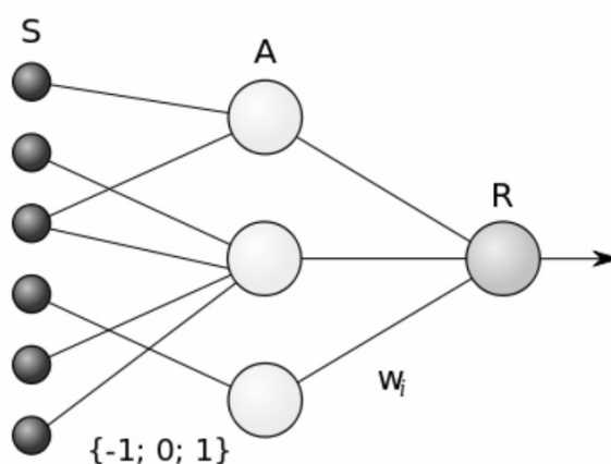
Рис. Пример архитектуры простейшей нейросети с внешними входами, где S-входные нейроны; А-скрытые нейроны, состоящие из одного или нескольких слоев; W-обучающие связи; R-выходные нейроны.
