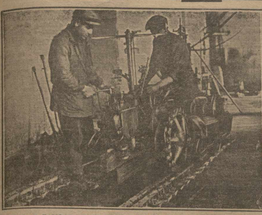
ТРАКТОР В РЕМОНТНОЙ МАСТЕРСКОЙ. Гусеничный трактор разобран до основания, — теперь можно приступать к замене изношенных частей.
