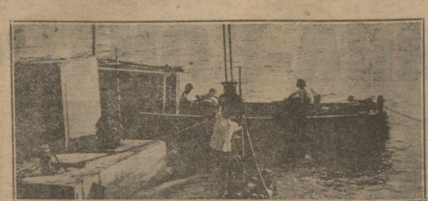
ПОТИ-ПОРТ. Установка подводного моста при помощи воллоза, ирана и т.д.
