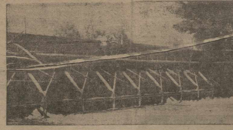
Головной шлюз Каравазской системы в действии. Вид со стороны камеры
