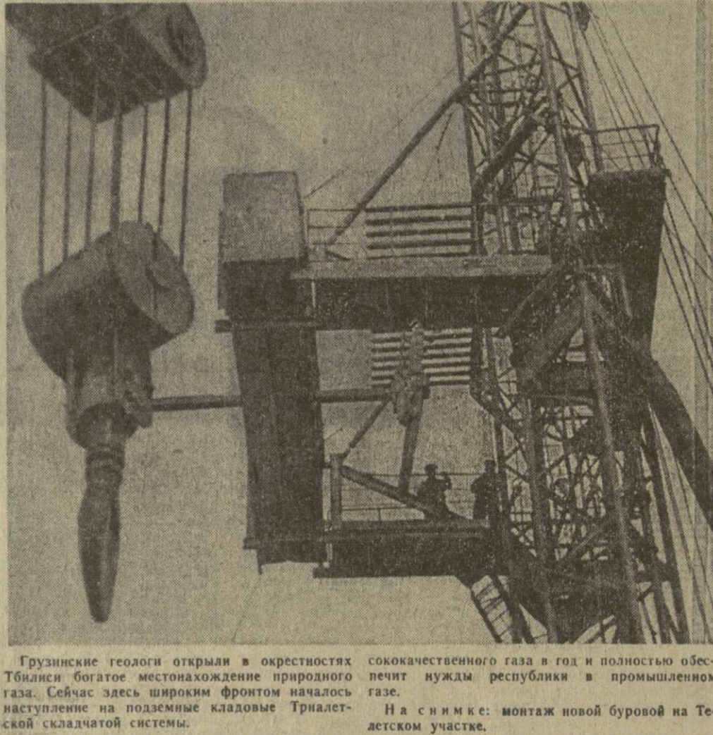
Грузинские геологи открыли в окрестностях Тбилиси богатое местонахождение природного газа. Сейчас здесь широким фронтом началось наступление на подземные кладовые Тrialetской складчатой системы.
