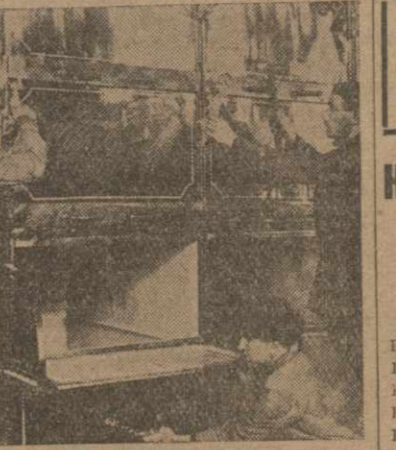
Завод № 1 Металлтреста Грузии принял крупный заказ на изготовление коносухи для Персии. На фото — сборка коносухи.
