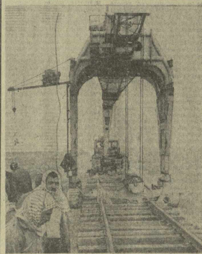
Сирийская Арабская Республика. На строительстве новой железной дороги Латакия — Алеппо — Камышли протяженностью 742 километра хорошо зарекомендовали себя советские путеукладчики, с помощью которых сирийские строители совместно с советскими инженерами и техниками прокладывают 1.500 метров железнодорожного пути за смену. На снимке: советский путеукладчик в действии. Фото К. Ампилова. (Фотохроника ТАСС).
