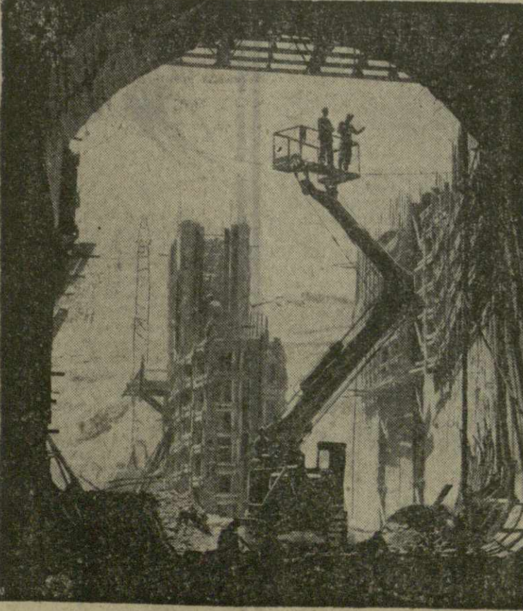
На снимке: сооружение тоннелей, по которым вода реки Или пойдет к турбинам Капчагайской ГЭС.
