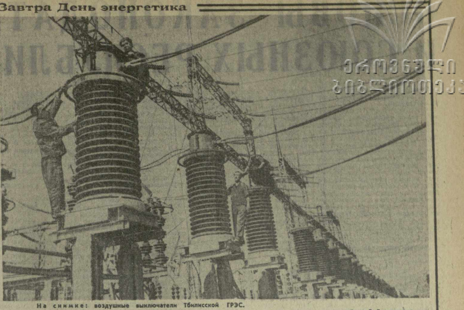
На снимке: воздушные выключатели Тбилисской ГРЭС. Фото Г. Вахтангадзе.
