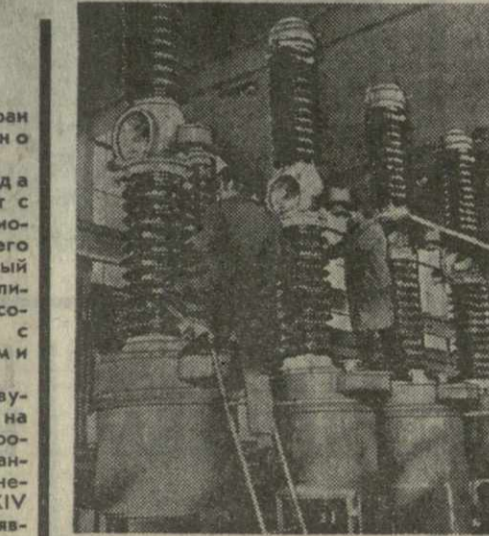
● СОЦИАЛИСТИЧЕСКАЯ ФЕДЕРАТИВНАЯ РЕСПУБЛИКА ЮГОСЛАВИЯ. В цехе электротехнического завода в Рипин близ Белграда. Продукция этого предприятия — трансформаторы, механические и масляные выключатели. Фото ТАНЮГ—ТАСС.
