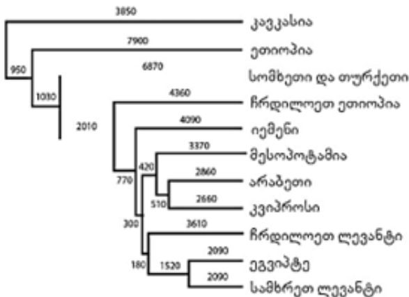
გრაფიკი. პოპულაციის გაყოფის დროის შეფასებები BATWING (Bayesian Analysis of Trees With Internal Node Generation) ახლო აღმოსავლეთის პოპულაციებისთვის, რომელიც გვიჩვენებს გაფართოების ისტორიას (a) J1, (b) J2 ჰაპლოჯგუფებისთვის. „Mapping Post-Glacial expansions: The Peopling of Southwest Asia.“ Daniel E. Platt et al. 2017. მიხედვით.
