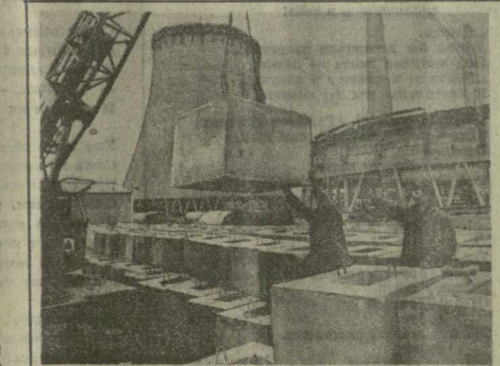
Чехословацкая. На самом востоке Словакии, там, где сливаются реки Лаборец и Уг, сооружается вторая очередь электростанции «Вонны». 12 турбоагрегатов электростанции, каждый по 110 мегаватт, будут вырабатывать 8 миллиардов киловатт-часов электроэнергии. Это больше, чем давали все электростанции Чехословакии в 1937 году.
