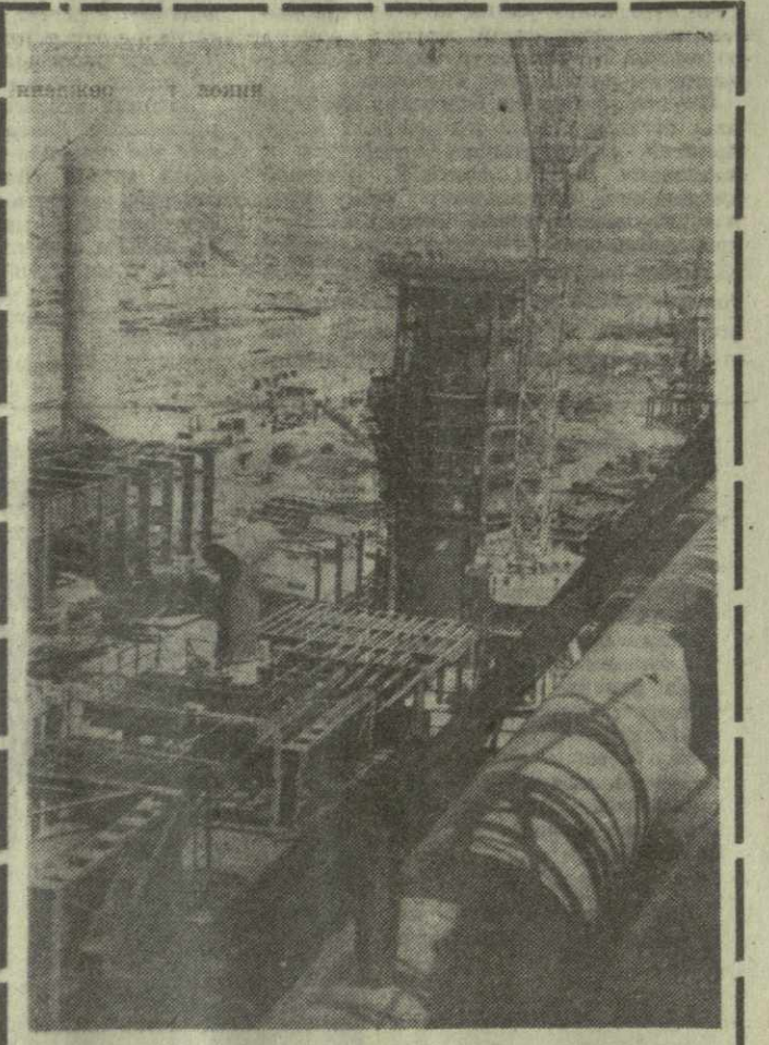
Индия. При техническом содействии и дружеской помощи Советского Союза в Бокоро (штат Бихар) сооружается крупнейший в Юго-Восточной Азии металлургический завод. На строительстве этого предприятия занято свыше 60 тысяч индийских рабочих, техников и инженеров. На стройке трудятся и советские специалисты. На снимке: первая домна. Ее строительство завершится осенью 1972 года. Фото Н. Кольцова. (Фотохроника ТАСС).
