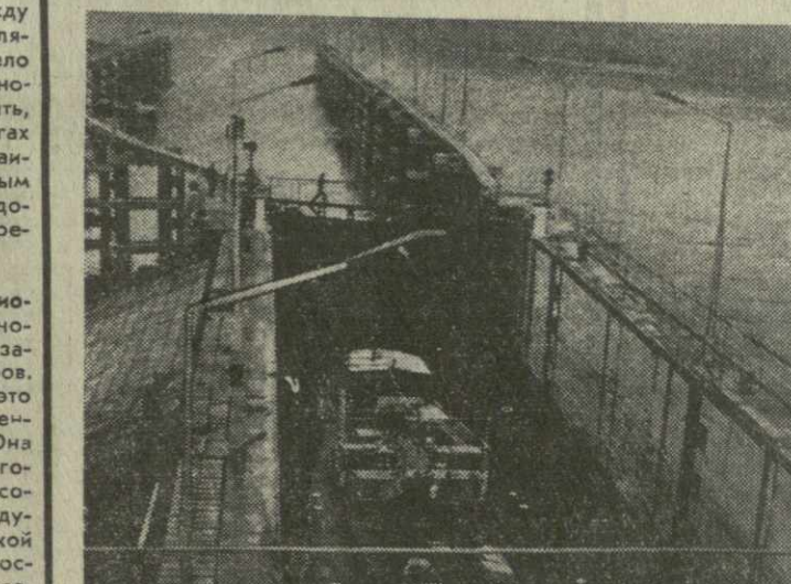
▲ ЮГОСЛАВИЯ. Завершено строительство крупнейшей в стране гидросистемы Дунай — Тиса — Дунай. Протяженность основных голубых магистралей этой системы 930 километров, обводнено благодаря им 500 тысяч гектаров пахотных земель. На снимке: один из шлюзов системы. (Фотохроника ТАСС).
