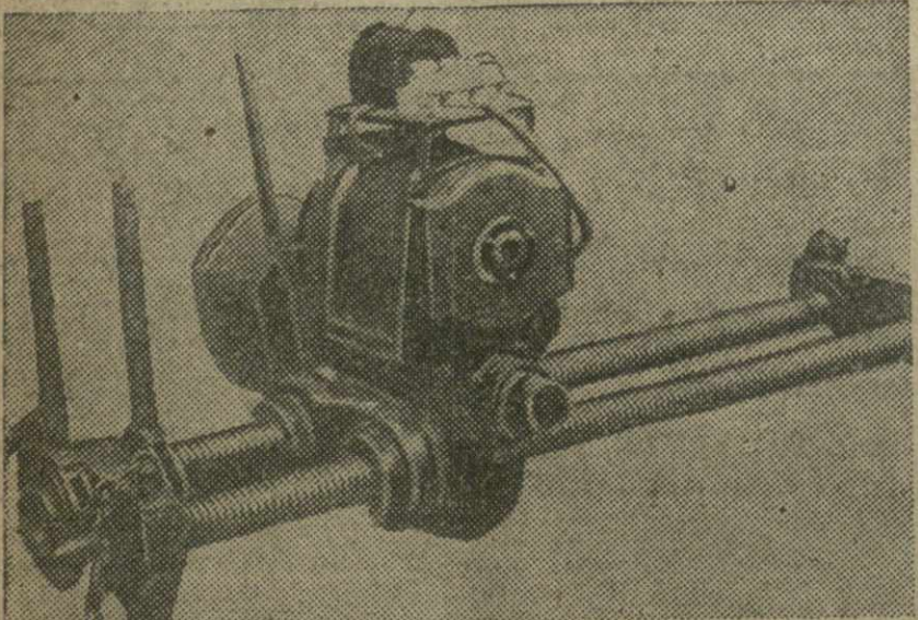
Установка для прокладки кабелей и труб без рытья траншей, через городские улицы, железнодорожные и трамвайные пути
