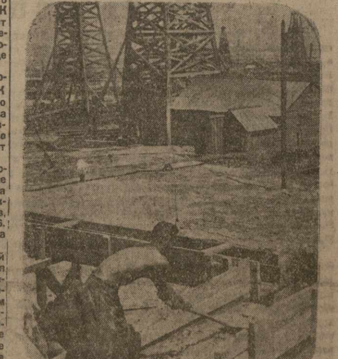
Промысел им. Микояна (Лок-Батан). Подготовка канав для циркуляции глинистого раствора на буровой № 43, пущенной в бурение в счет «300».
