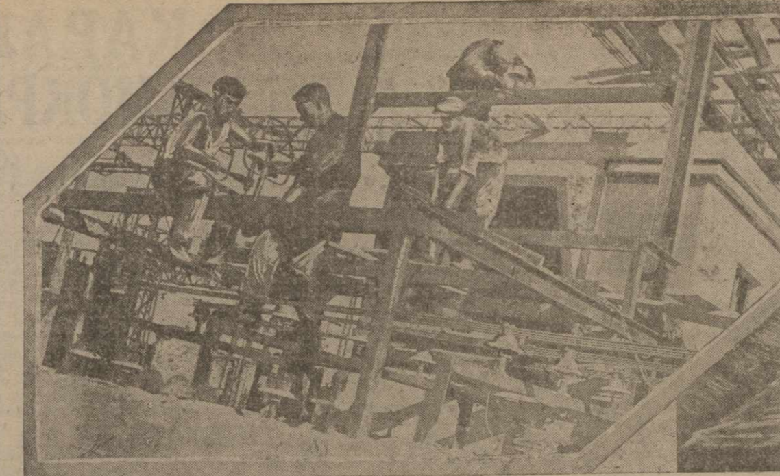
На снимке: монтаж водяного ротора для нагрузки генератора и главный канал
