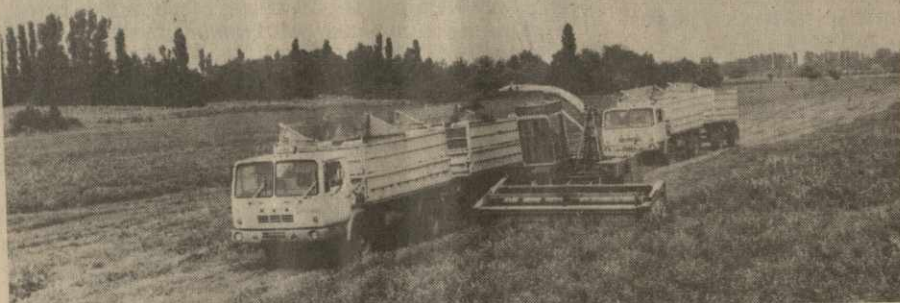
Коллектив Кутаисского ордена Трудового Красного Знамени автомобильного завода имени С. Орджоникидзе готовится к серийному производству автопоездов сельскохозяйственного назначения «КАЗ-4540». В четвертом году пятилетки сельское хозяйство страны получит 20 тысяч таких автопоездов.
