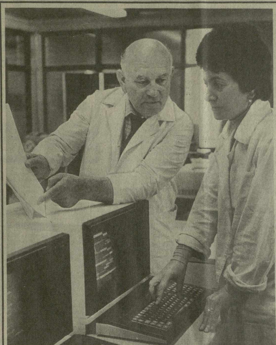
Система оперативного диспетчерского управления разработана и внедрена коллективом руставского научно-производственного объединения «Автоматром» на руднике Ахали-Итхвски имени З. А. Патаридзе ПО «Чхатурмарганец».
