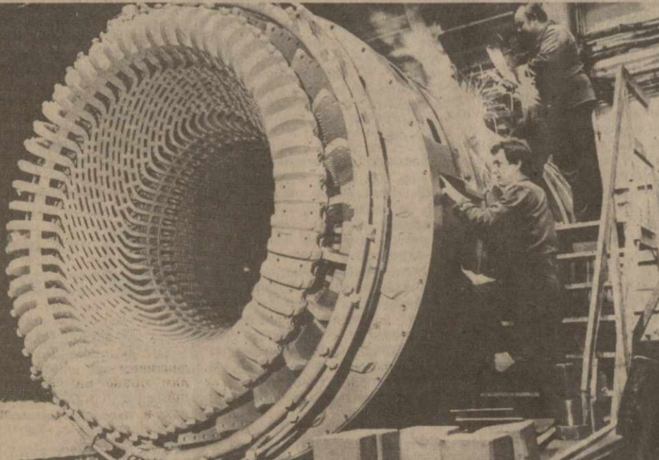
● СССР. Комбинат «Шкода» имени В. И. Ленина в городе Пльзень участвует в осуществлении более 20 программ в рамках социалистической экономической интеграции, прежде всего в области энергетики. На с н и м к е: в цехе предприятия.
