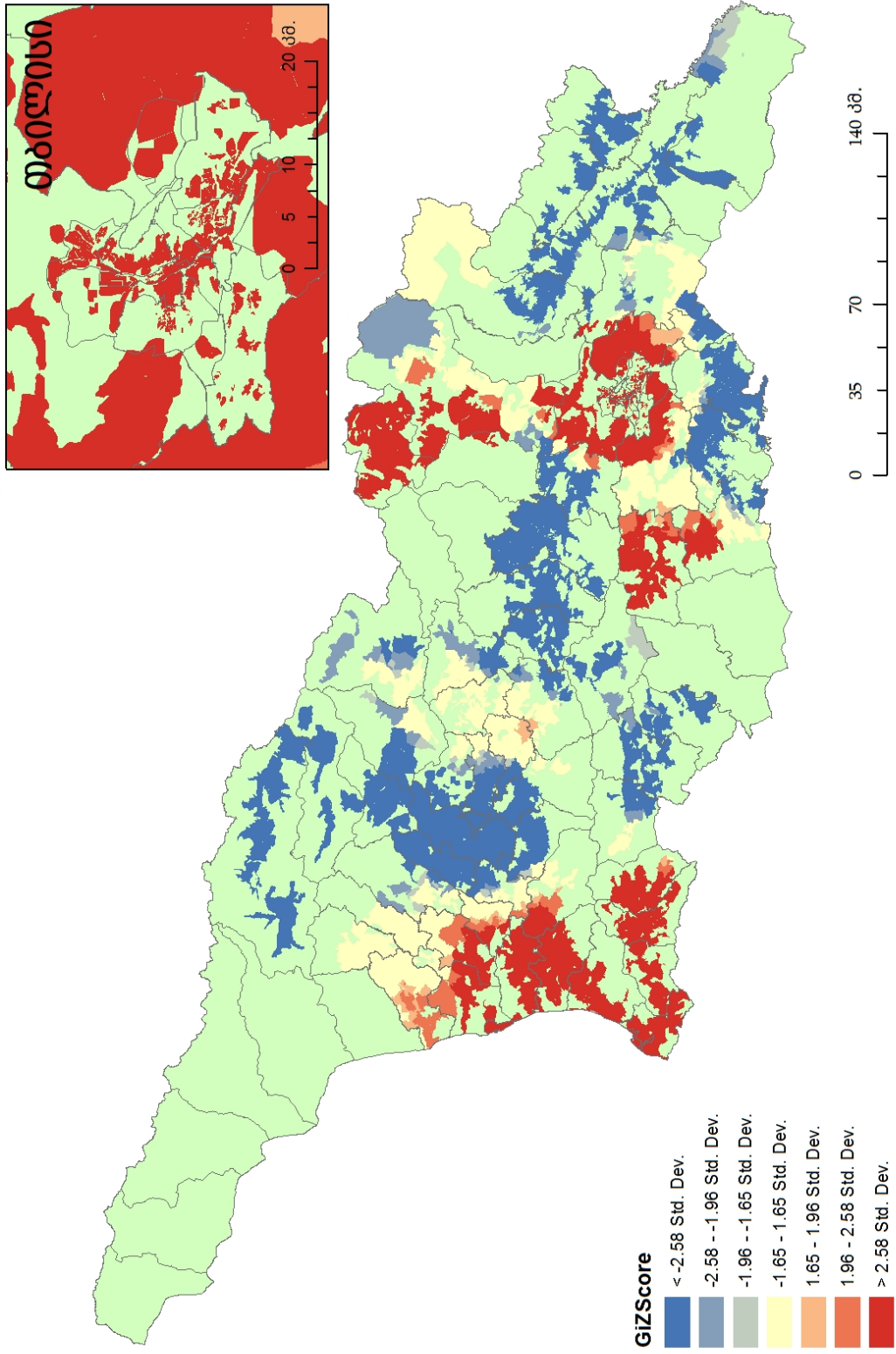
დანართი დ.9. 2010 წლის მუნიციპალური არჩევნები. „ერთიანი საბჭოს“ ხმების სივრცითი აგტოკორელაციის ადგილობრივი მაჩვენებელი (ჯეითის-ორდის G* კოეფიციენტი)
