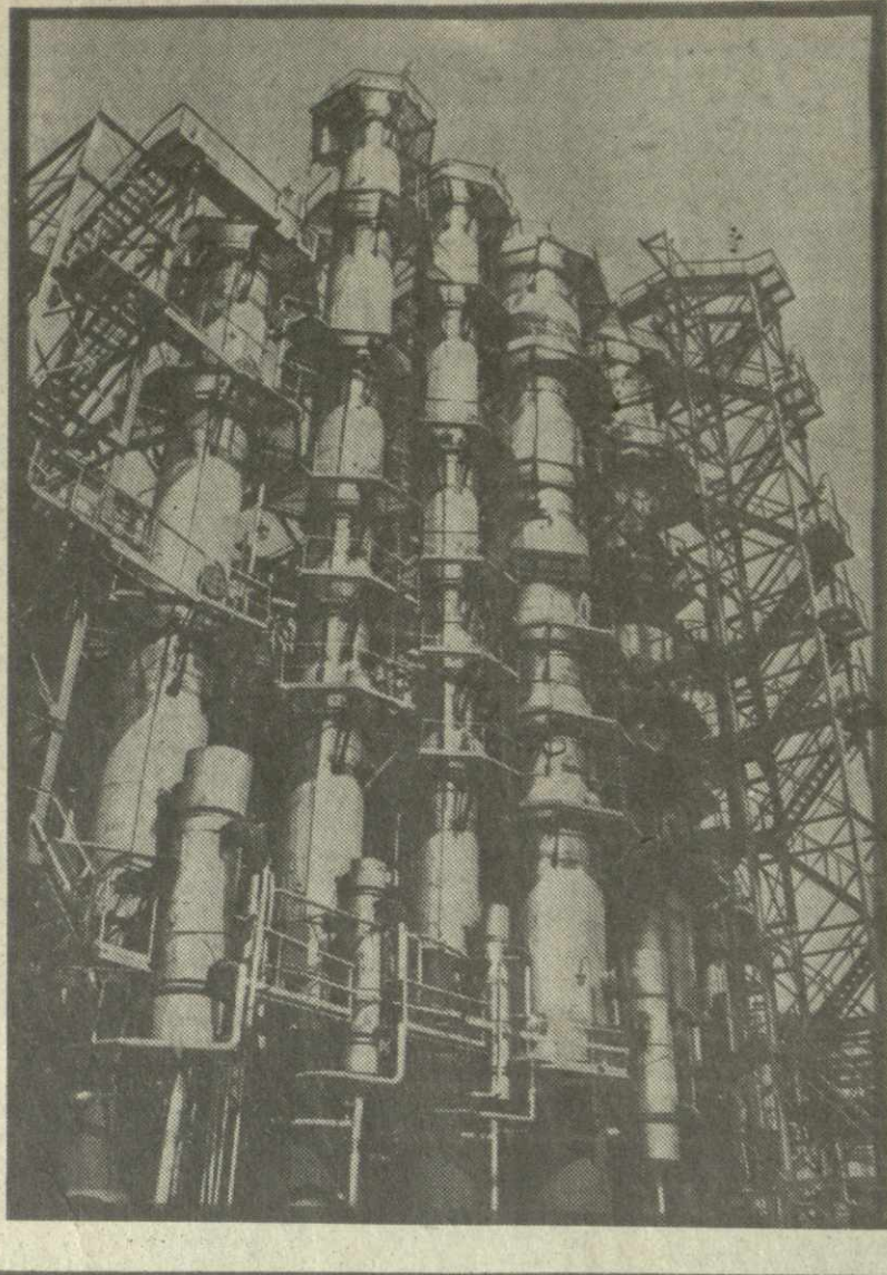
УСТАНОВКА для получения водорода из огромных газов американской фирмы «Менсифа», которую обслуживает всего один оператор, введена в эксплуатацию в руставском научно-производственном объединении «Азот». Ежегодный экономический эффект — 5 миллионов рублей при затратах на приобретение и установку оборудования в два миллиона долларов. Но самое главное — новая техника экологически чиста.
