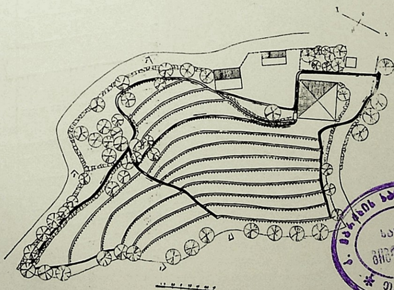
სურ. 1. ზ. არაბელაძის საკარმიდამო ნაკვეთის მორწყვის სისტემის კრილი და გეგმა (სოფ. ბელლეთი)
