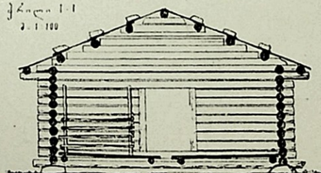
სურ. 4. ძირითადი ჯარგვალი (ახალდაბის საძვრები)
