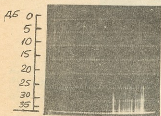
Рис.2-3. Момент фрикации интервокальной афр. zh в слове zhīzhì. Дикт. 2.
