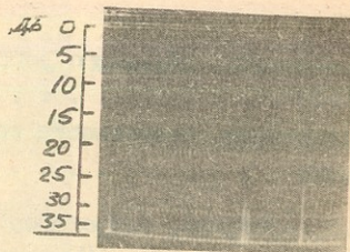
Рис.2-7. Момент начала фрикации интервокальной афр. zh в слове qīzha. Дикт.1.
