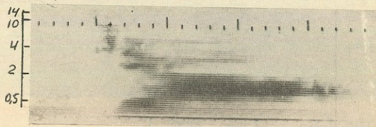
Рис. I-1. zha. в первом тоне. Дикт. 2.
